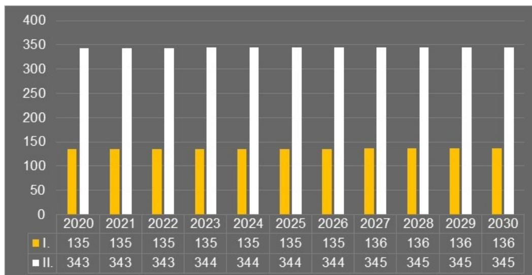
Tabuľka č. 2 : Prehľad spotreby Slovenska na nasledujúcich 10 rokov
